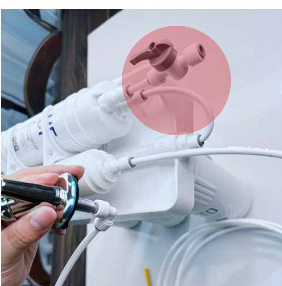
Свържете 1/4" пластмасов сферичен кран
